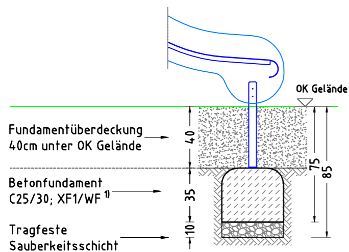
FUNDAMENTSCHNITT(E) M 1:25
