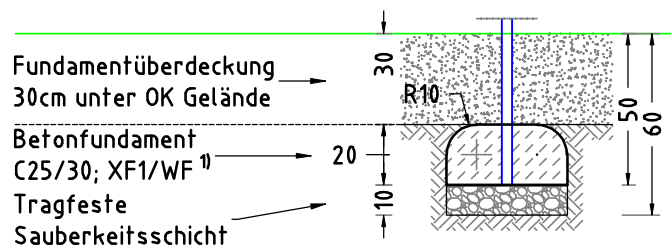
FUNDAMENTSCHNITT(E) M 1:25
